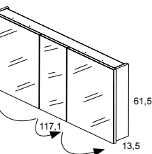
Camerino 120 3P BINOVA-NIKA F-13,5 / BINOVA-NIKA cupboard 120 3D D-13,5
